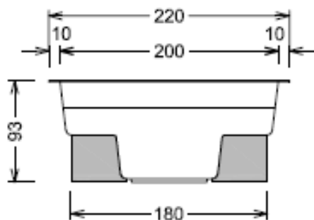
Ansicht Skimmerseite
