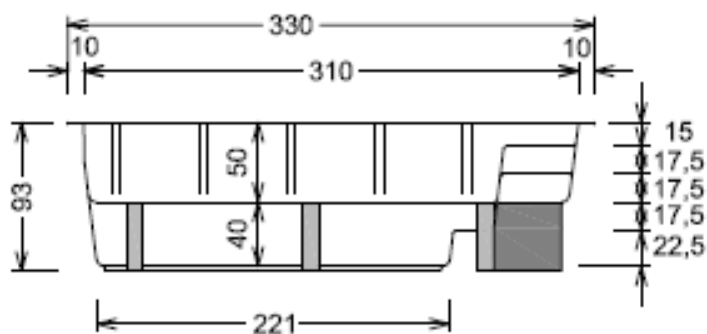
Seitenansicht
