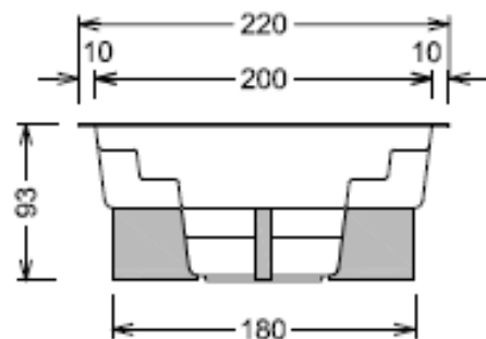
Ansicht Treppenseite
