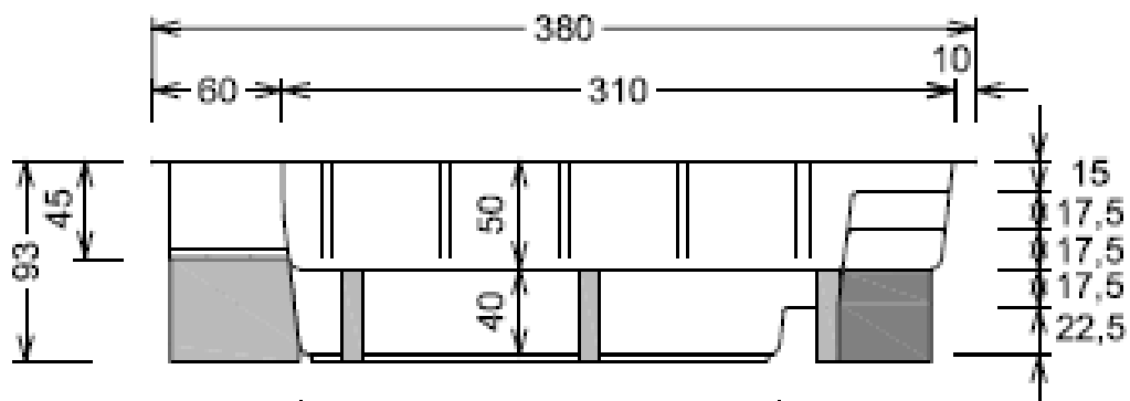
Ansicht Skimmerseite
