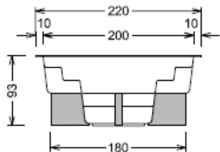
Ansicht Treppenseite
