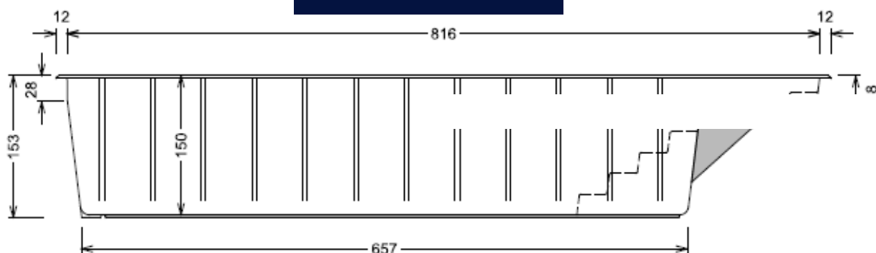
Seitenansicht
