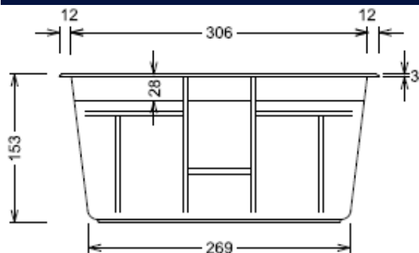
Ansicht Skimmerseite
