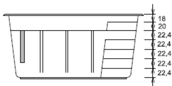
Ansicht Treppenseite
