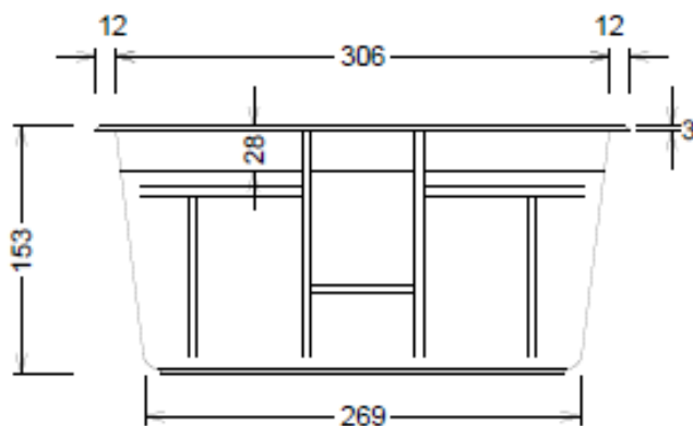
Ansicht Skimmerseite
