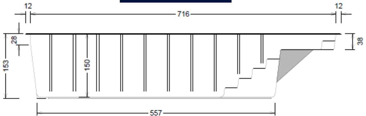
Seitenansicht
