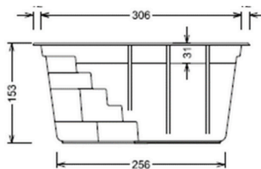
Ansicht Treppenseite
