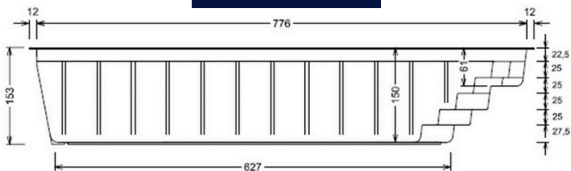
Seitenansicht
