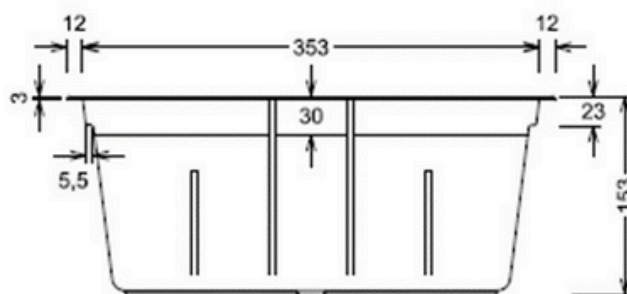
Ansicht Skimmerseite
