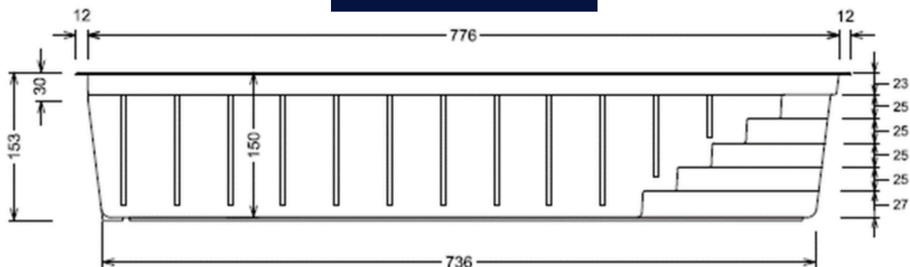
Seitenansicht
