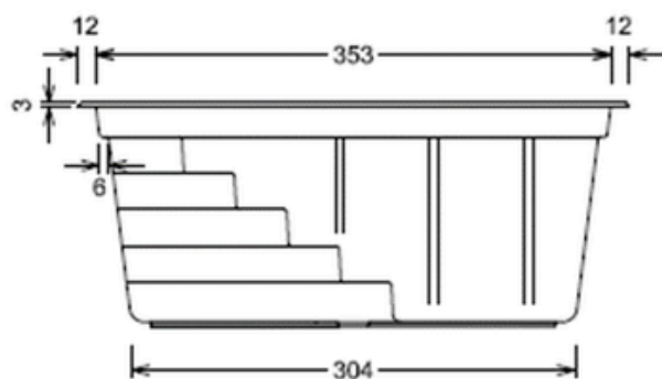
Ansicht Treppenseite
