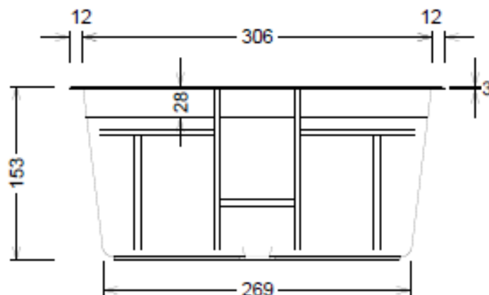
Ansicht Skimmerseite
