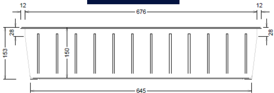
Seitenansicht
