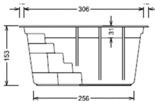
Ansicht Treppenseite
