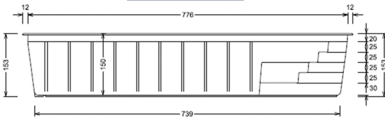
Seitenansicht
