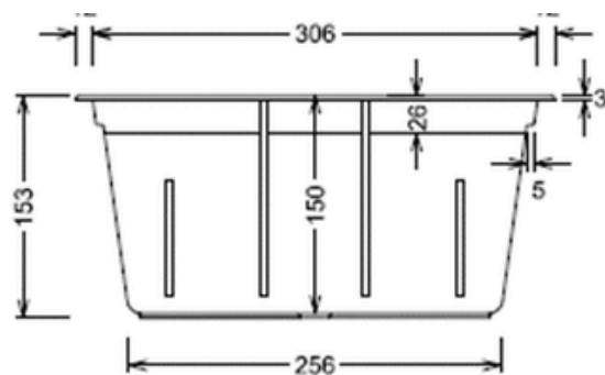
Ansicht Skimmerseite
