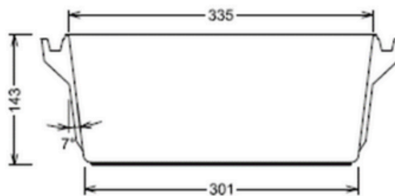
Querschnitt
