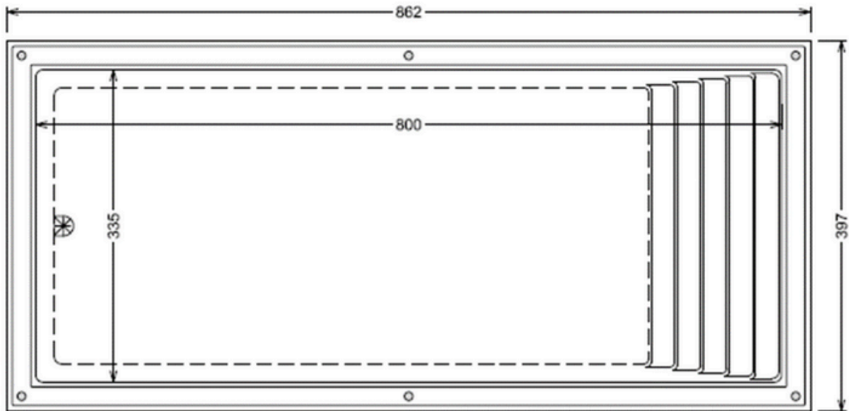
Grundriss
