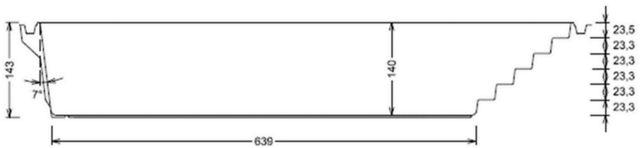
Seitenansicht
