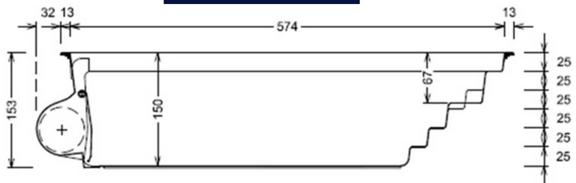
Ansicht Skimmerseite
