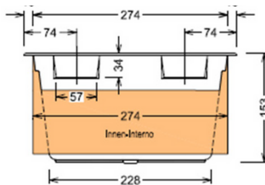
Ansicht Skimmerseite
