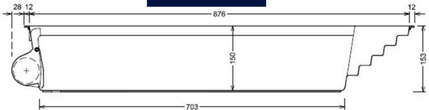
Seitenansicht
