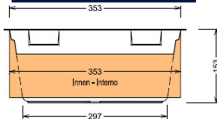
Ansicht Skimmerseite
