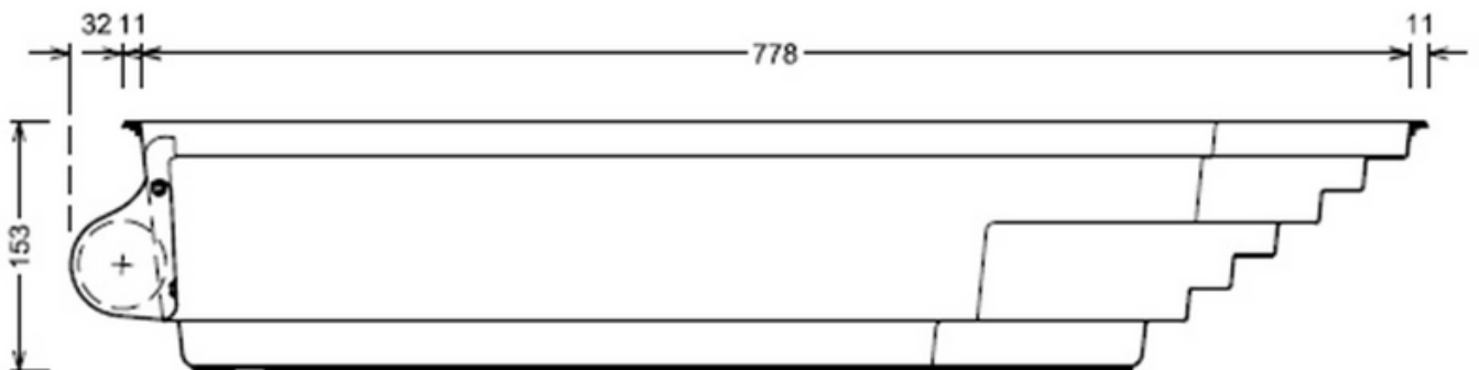
Ansicht Skimmerseite
