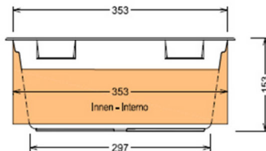
Ansicht Skimmerseite
