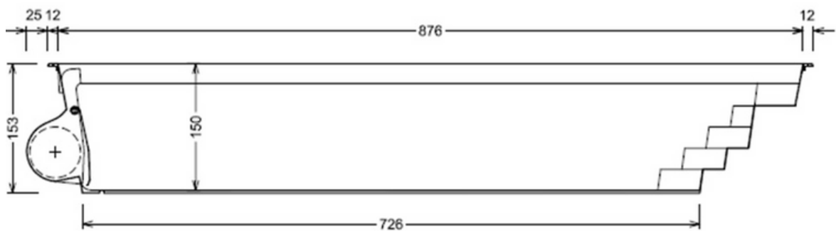
Ansicht Skimmerseite
