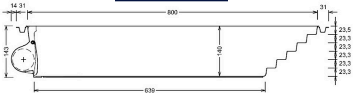
Seitenansicht
