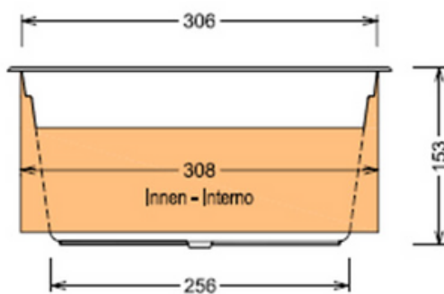
Ansicht Skimmerseite
