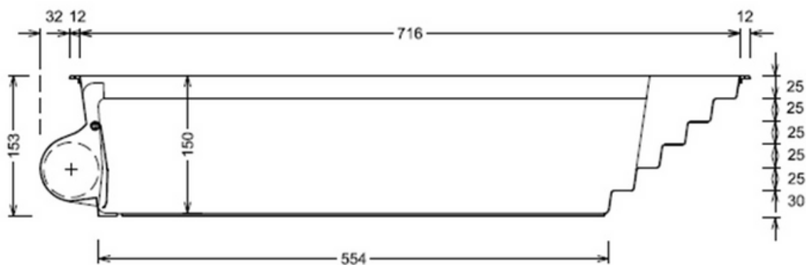
Ansicht Skimmerseite
