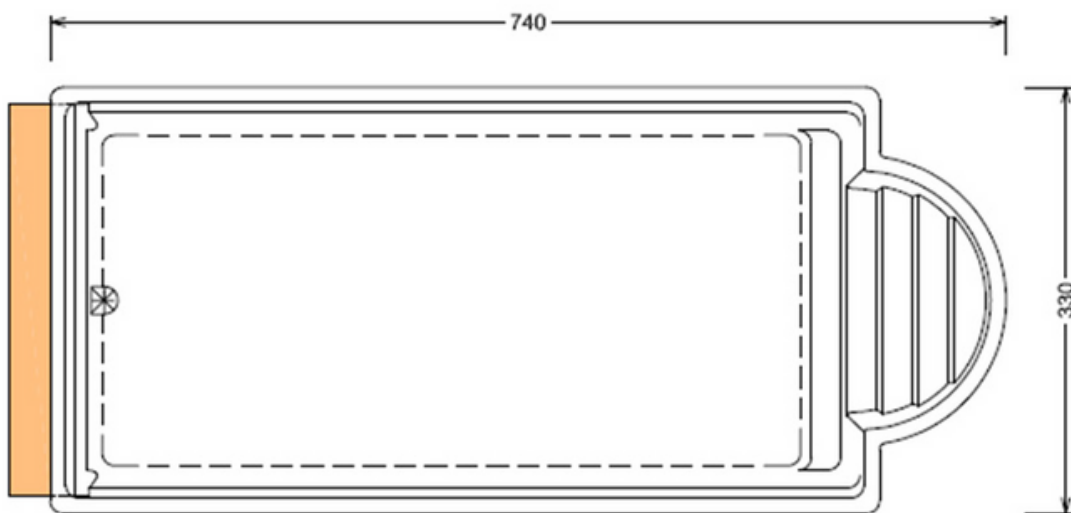
Seitenansicht
