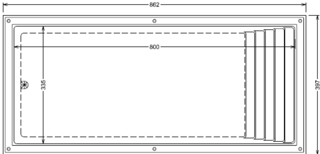
Grundriss
