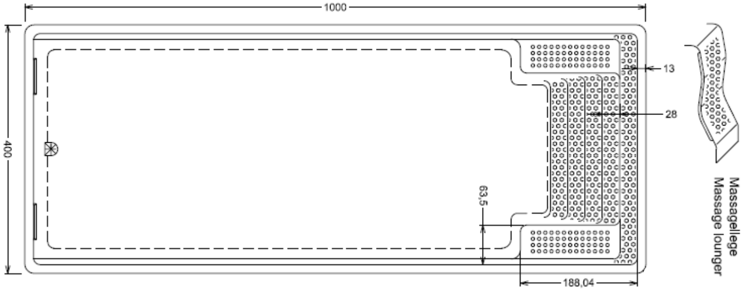
Grundriss
