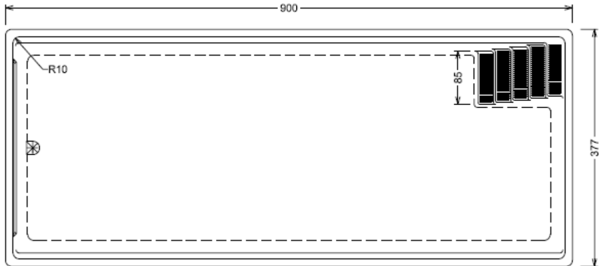
Grundriss
