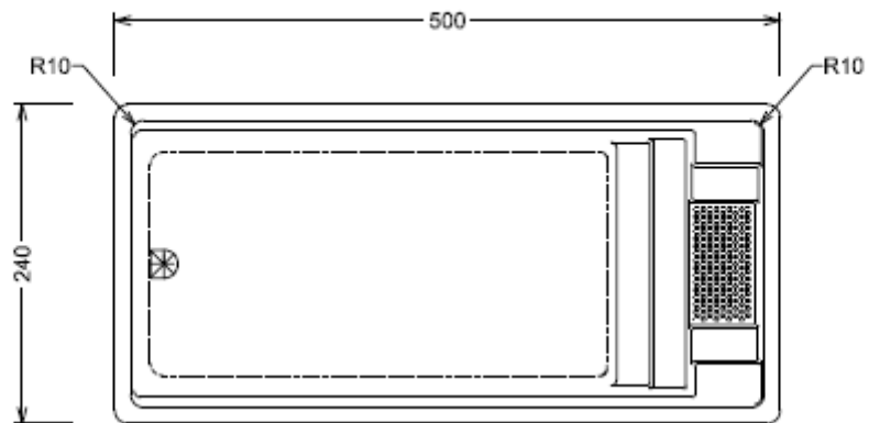
Grundriss
